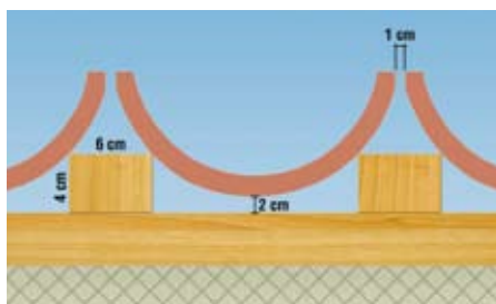
Fig. 2: I coppi dovranno poggiare sui fianchi, senza toccare il listello inferiore (almeno 2 cm di distanza) e senza toccarsi tra loro (circa 1 cm di distanza). Fig. 2: Concave tiles must rest on their sides without touching the bottom batten (at least 2 cm away) and without touching one another (distance approx. 1 cm).
