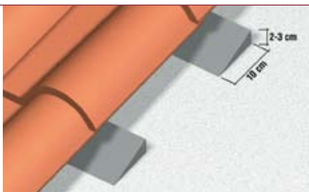
Fig. 5: Dimensioni "tipo" dell'elemento di supporto (cordolo di malta preconstituito) delle tegole. Fig. 5: "Typical" dimensions of the tile support element (pre-cast composition mortar fillet).
