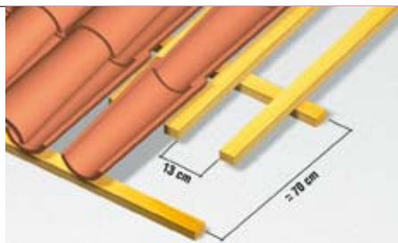
Fig. 1: La messa in opera dei coppi deve essere eseguita esclusivamente su una doppia listellatura. Fig. 1: Concave tiles may only be laid on a double batten framework.
