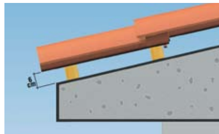
Fig. 4: Per mantenere la stessa inclinazione del resto del manto, le tegole della prima fila dovranno poggiare su un listello più alto di due centimetri rispetto agli altri. Fig. 4: To maintain the same pitch as the rest of the roof covering, the tiles on the first row should be placed on batten strips that are two centimetres higher than the others.
