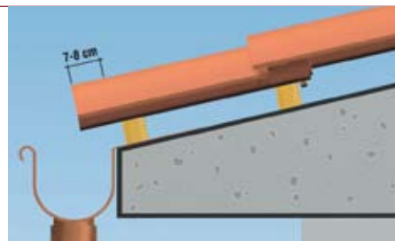
Fig. 3: La sporgenza delle tegole della prima fila sul canale di gronda deve essere circa un terzo del diametro della gronda stessa. Fig. 3: The first row of tiles must project over the guttering for about one third of the width of the gutter itself.
