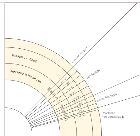
Fig. 6: Queste indicazioni possono variare in funzione dell'esposizione del tetto e della lunghezza di falda. Oltre il 45% di pendenza la fila di gronda va sempre fissata. Fig. 6: These guidelines may vary according to the exposure of the roof and the length of the pitch. If the slope is greater than 45%, then the eaves course must always be fixed into place.
