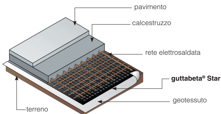
Fig. 2 Posa orizzontale
