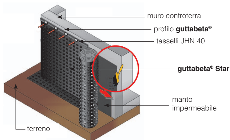
Fig. 1 Posa verticale
